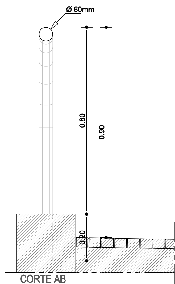
Pormenor de Guardas
