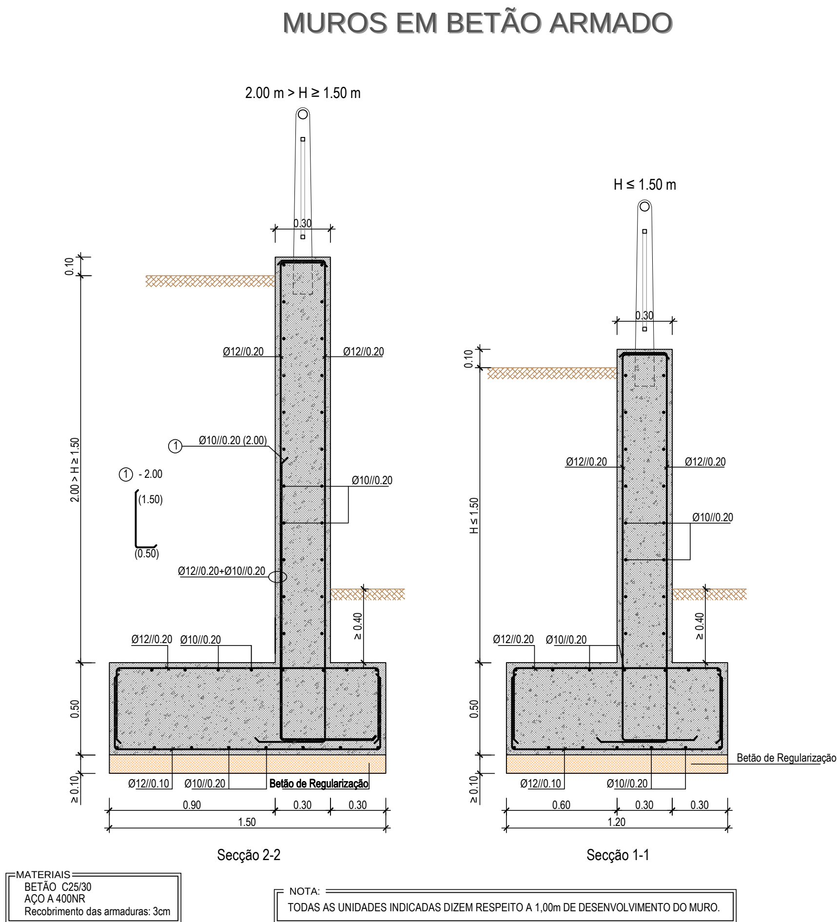
Muro de Suporte - Pormenor
