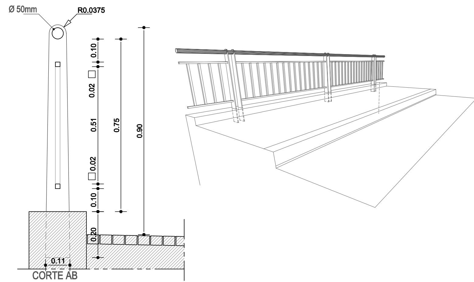
Pormenor de Gradeamentos
