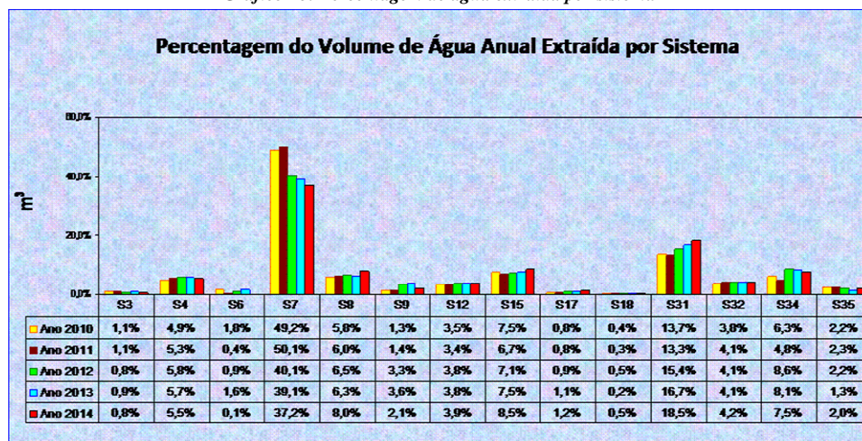
Gráfico 26: Percentagem de água extraída por sistema
