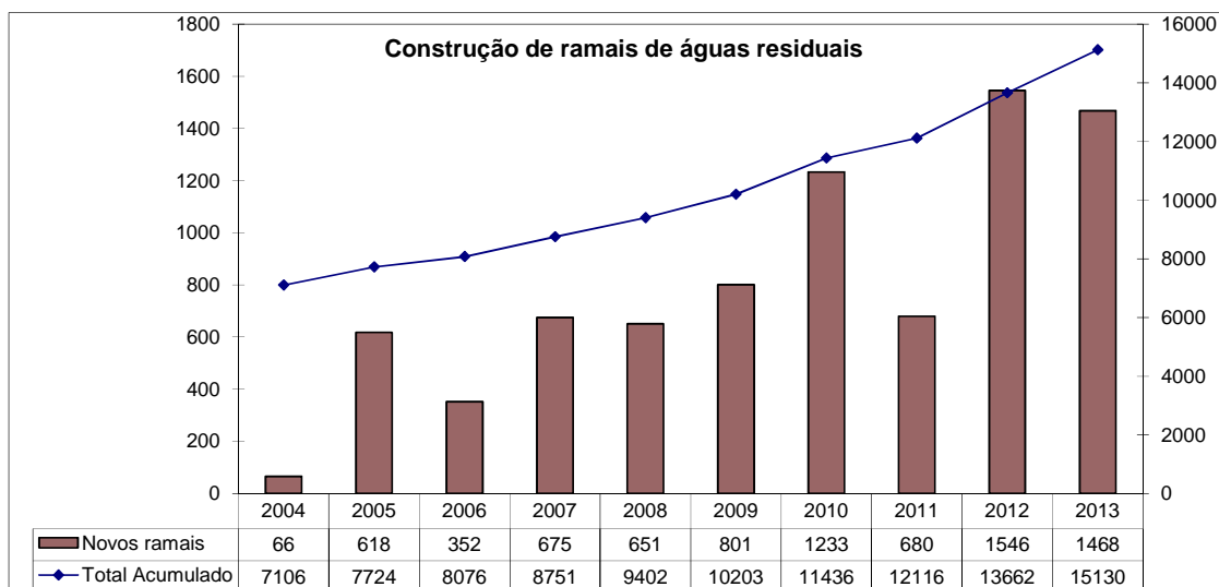
Gráfico 32 – Construção de ramais de águas residuais
