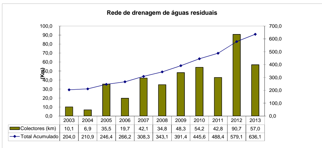
Gráfico 29 – Evolução da construção de Rede de Saneamento no Concelho
