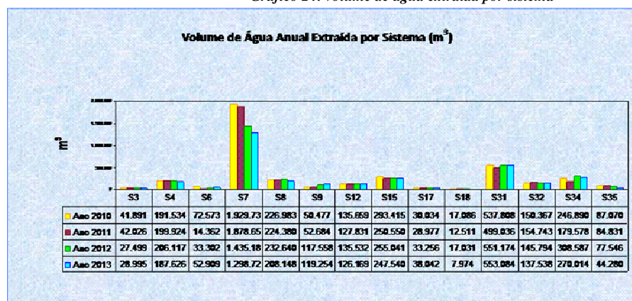
Gráfico 24: volume de água extraída por sistema
