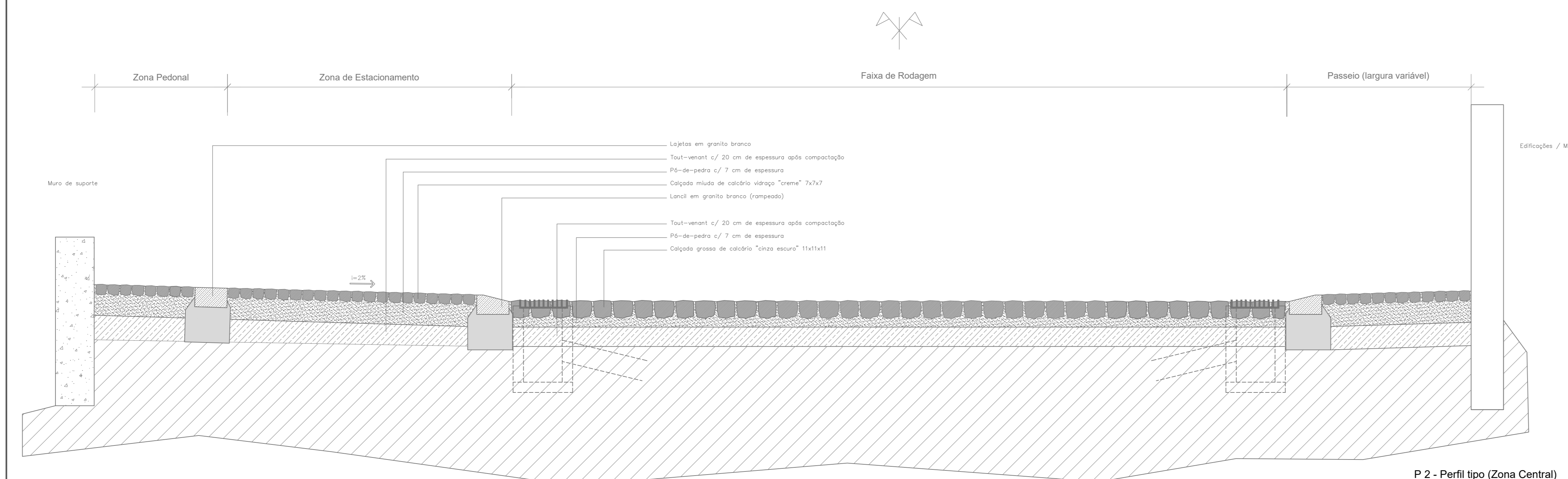
P 2 - Perfil tipo (Zona Central) (Data horizontal)
