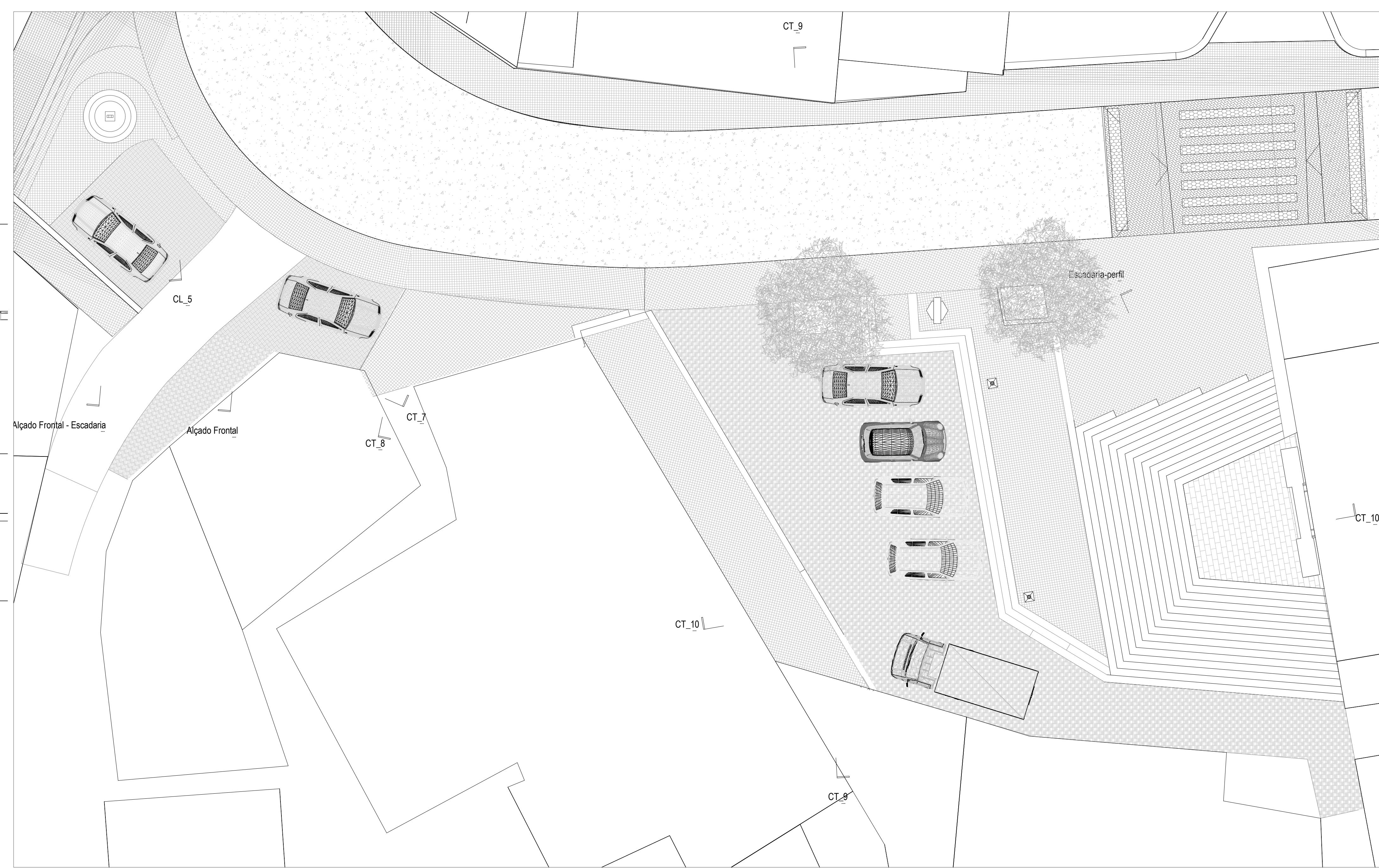
Planta do largo da Igreja (novo)
